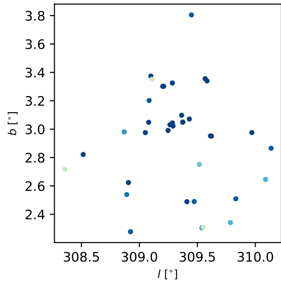
Platais 10
