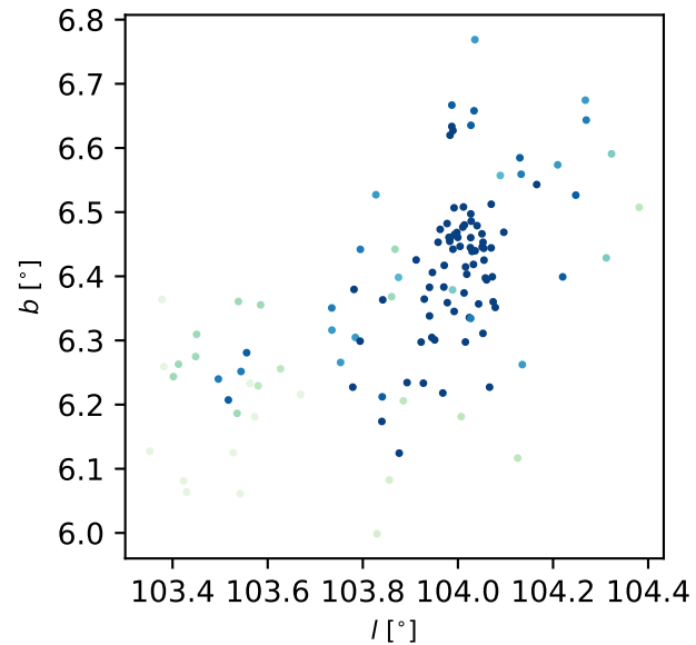
NGC 7160
