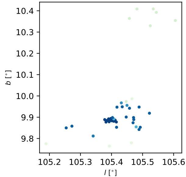
NGC 7129
