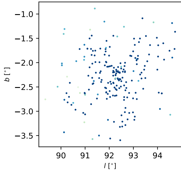
NGC 7092
