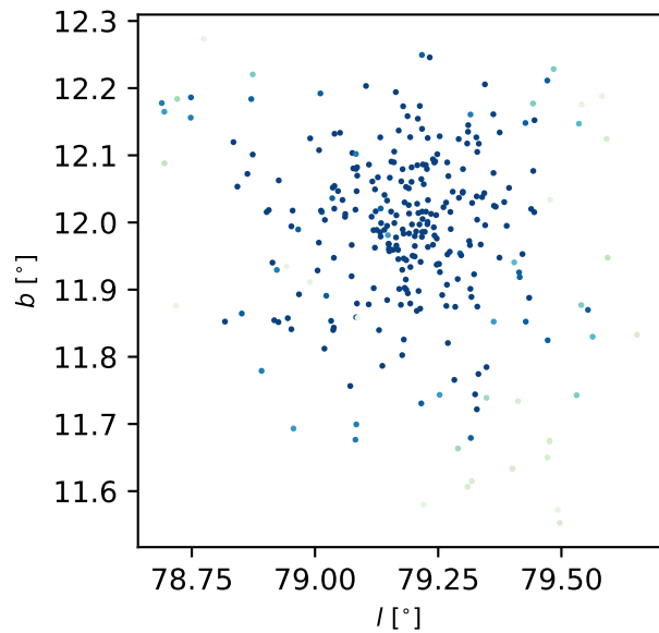
NGC 6811
