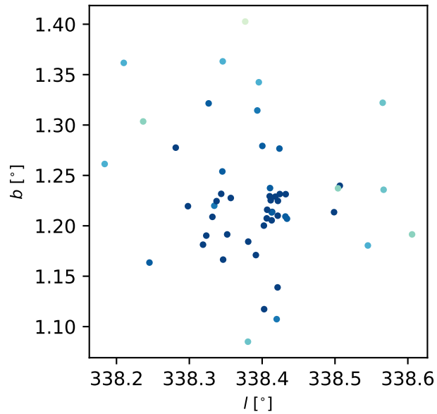
NGC 6178
