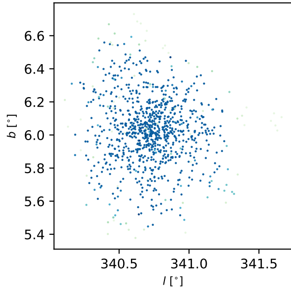
NGC 6124
