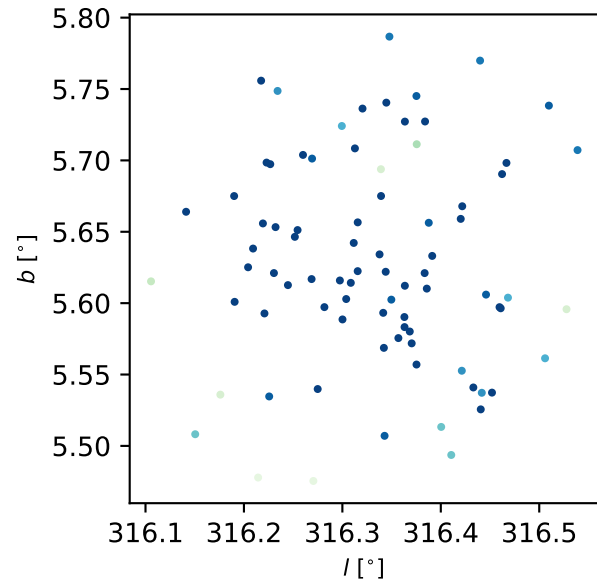
NGC 5593
