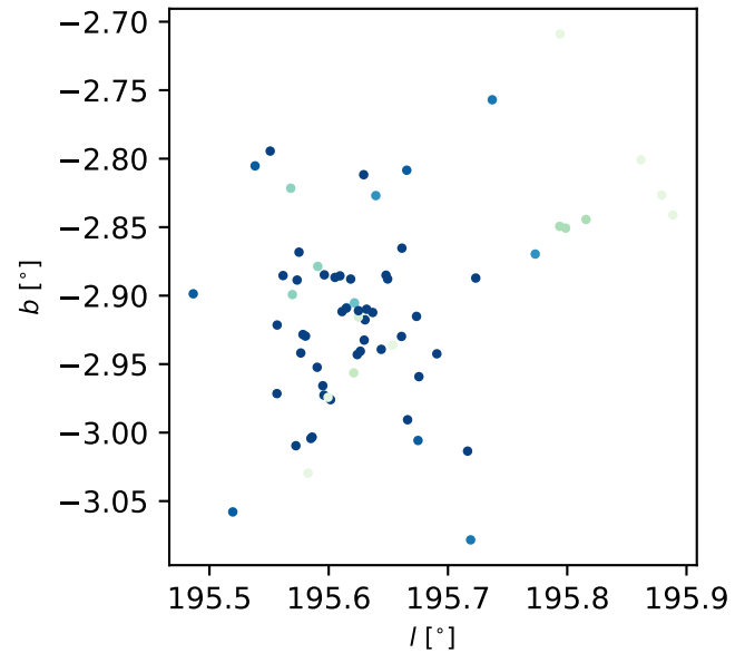
NGC 2169
