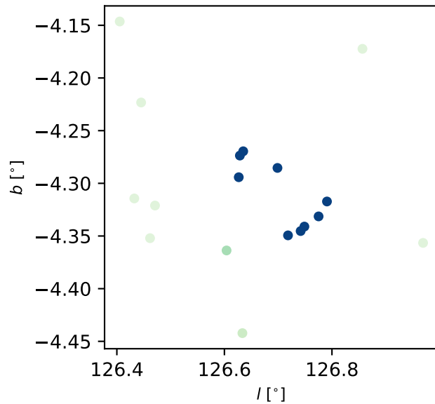
NGC 457
