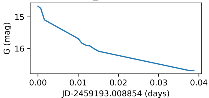
Star16_GWAC171126A
