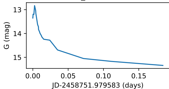
Star160_GWAC190925A
