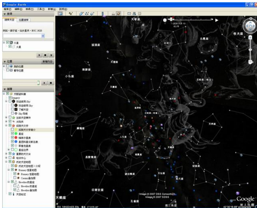
图 5GS 中显示的 Hevelius 星座图
