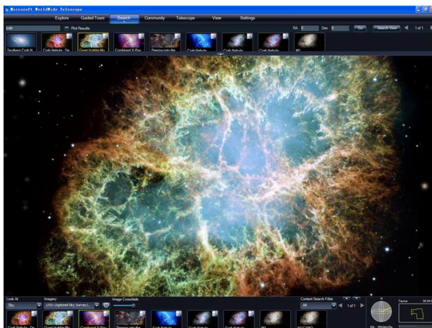
压题图：功能强大、界面华丽的 WWT
