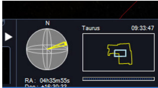
图 3 WWT 界面右下角显示当前浏览位置的天球投影和星座位置
