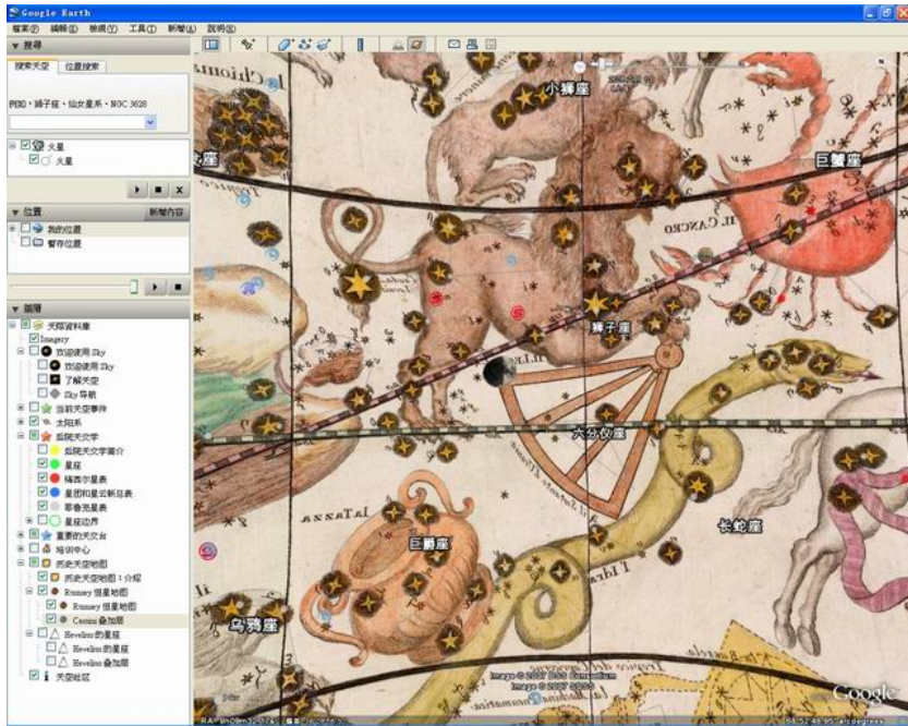
图 4GS 中显示的 Rumsey Cassini 古星图
