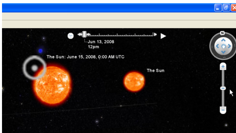
图 6GS 中的时间游标
